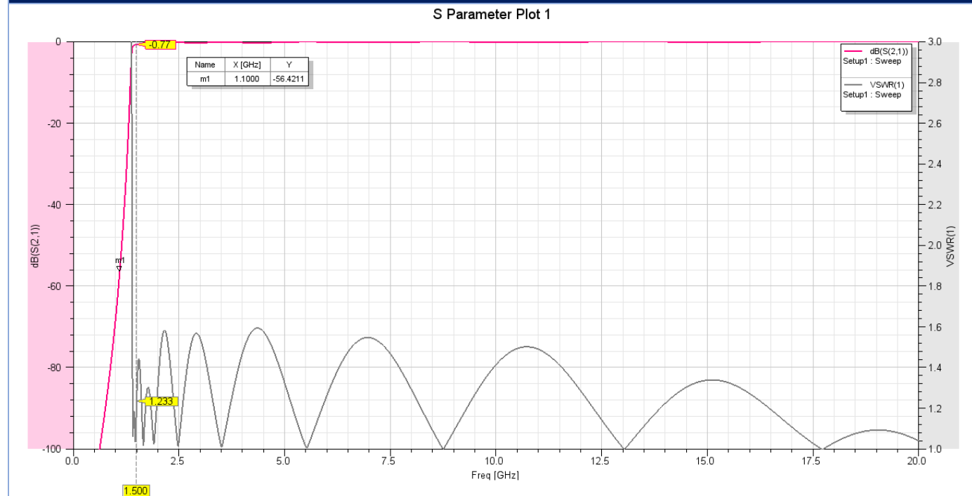
S Parameter Plot 1
