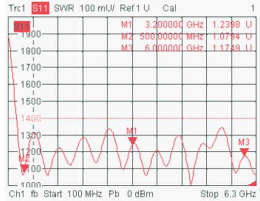
Input VSWR
